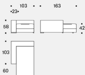
Penisola Fissa DX-SX 163 / Fixed right-left chaise longue 163 / 23
